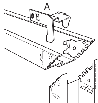
Verstekverbindingsbeugel
