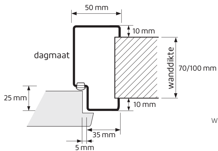
Profiel opdekuitvoering
