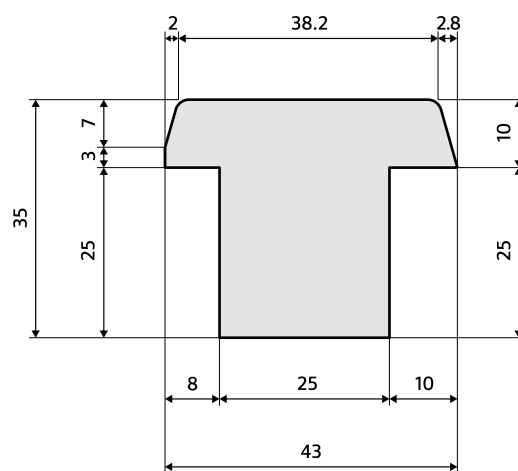
Tongnaald voor dubbele opdekdeuren
