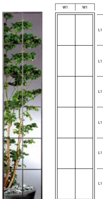
W1 en L1 variëren per glasmaat
