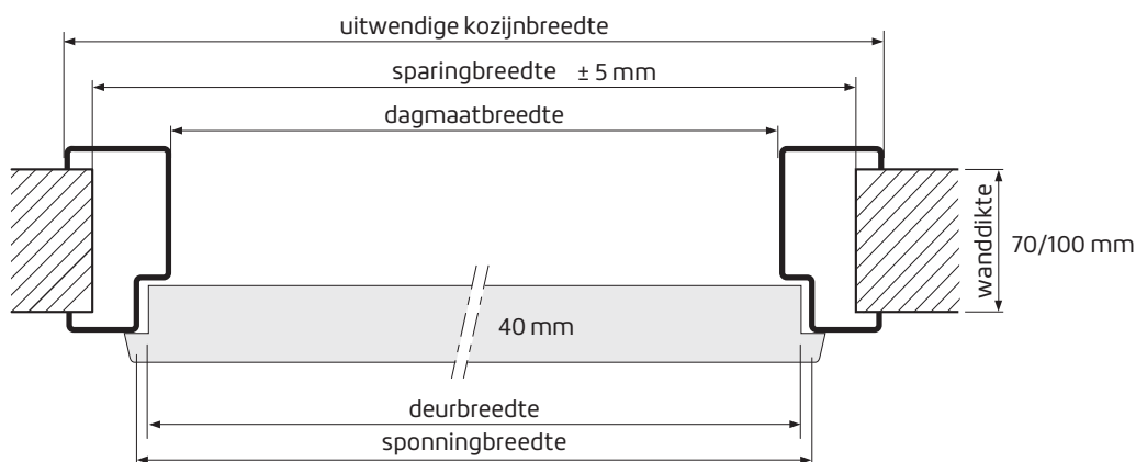
Horizontale doorsnede opdekuitvoering
