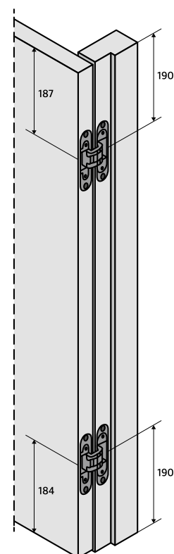
KUBICA (blinde) scharnieren. Vaste maten scharnierinkrozing.
